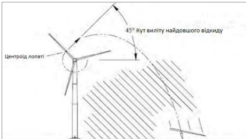
Рис. 7.1. Відрив лопаті вітроагрегата
